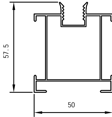
Mellemstolpe profil
