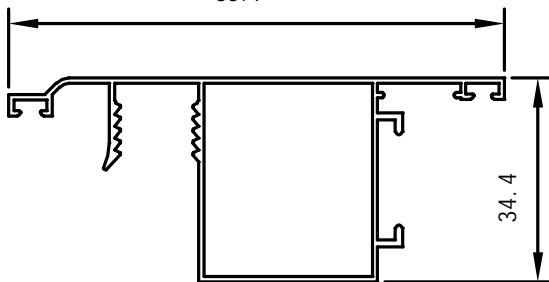
Vinduesramme profil
