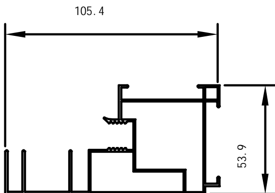
Sokkel profil
